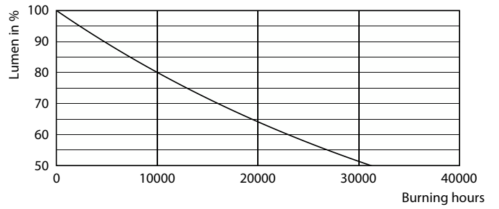
Lumen Maintenance Diagram - 9A19/CNG/850/FR/P/E26/ND 4/1CT
